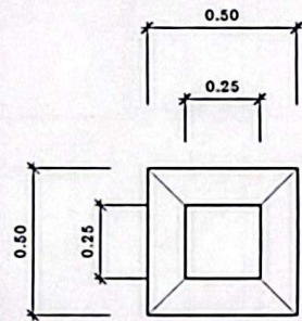
ฐานโคมไฟ คสล.
