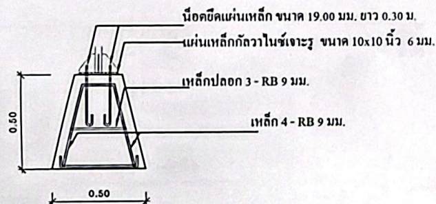
แบบขยายฐานโคมไฟ
