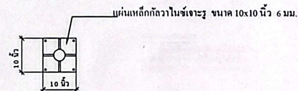
แผ่นเหล็กยึดเสาโคมไฟ
